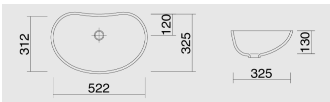
FONTANA FD-520 522 x 325 x 130 mm
